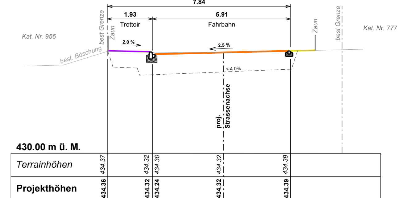
Profil 11 144.30m
