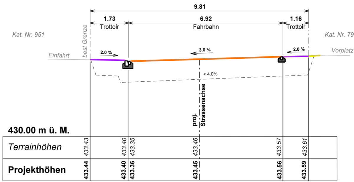
Profil 3 14.00m
