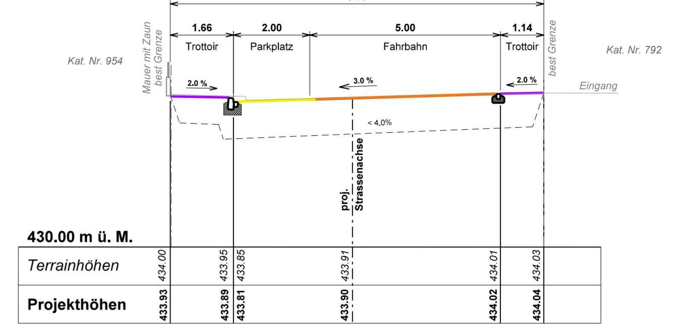
Profil 7 80.00m
