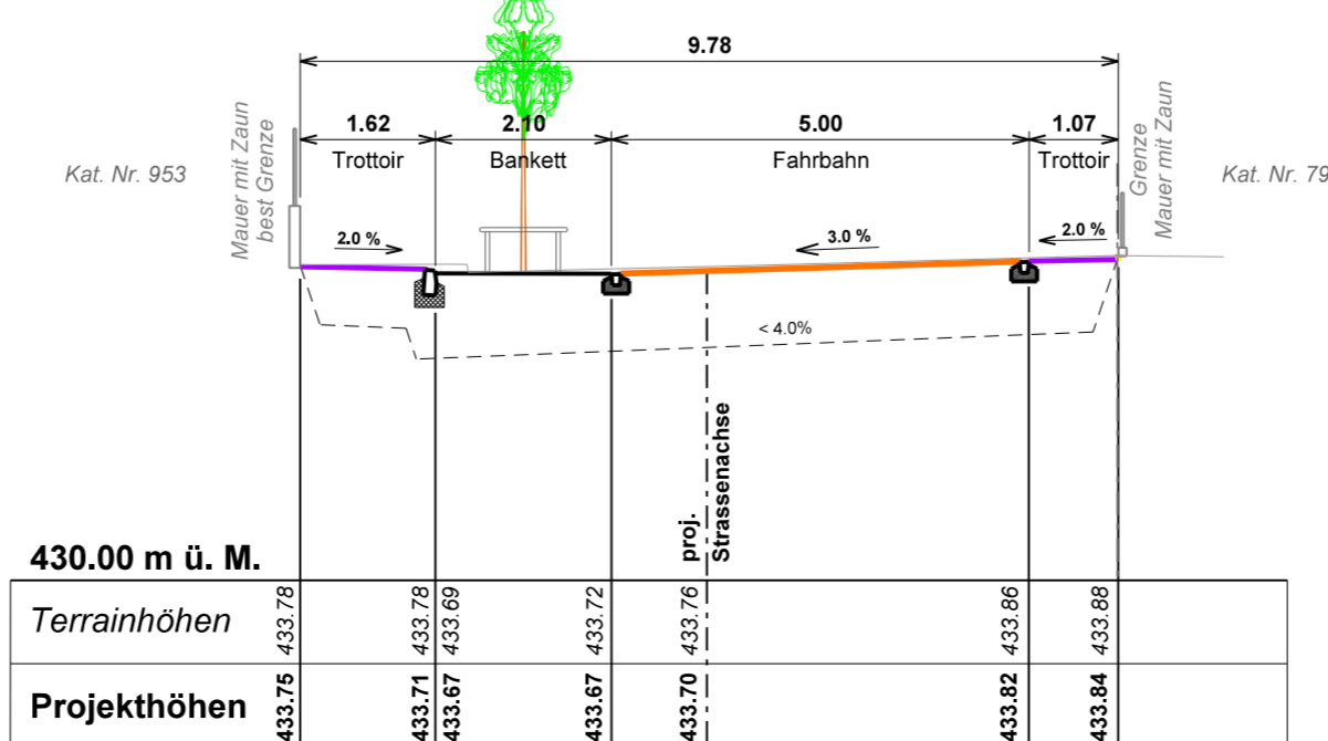
Profil 6 55.00m
