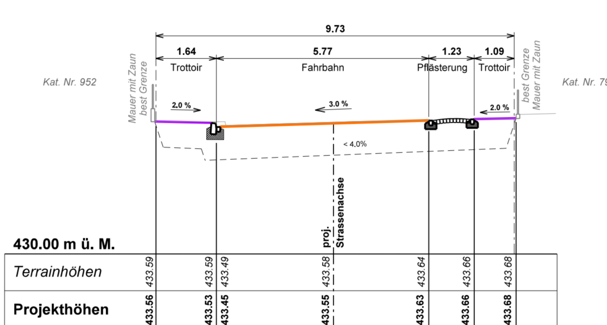
Profil 4 30.00m
