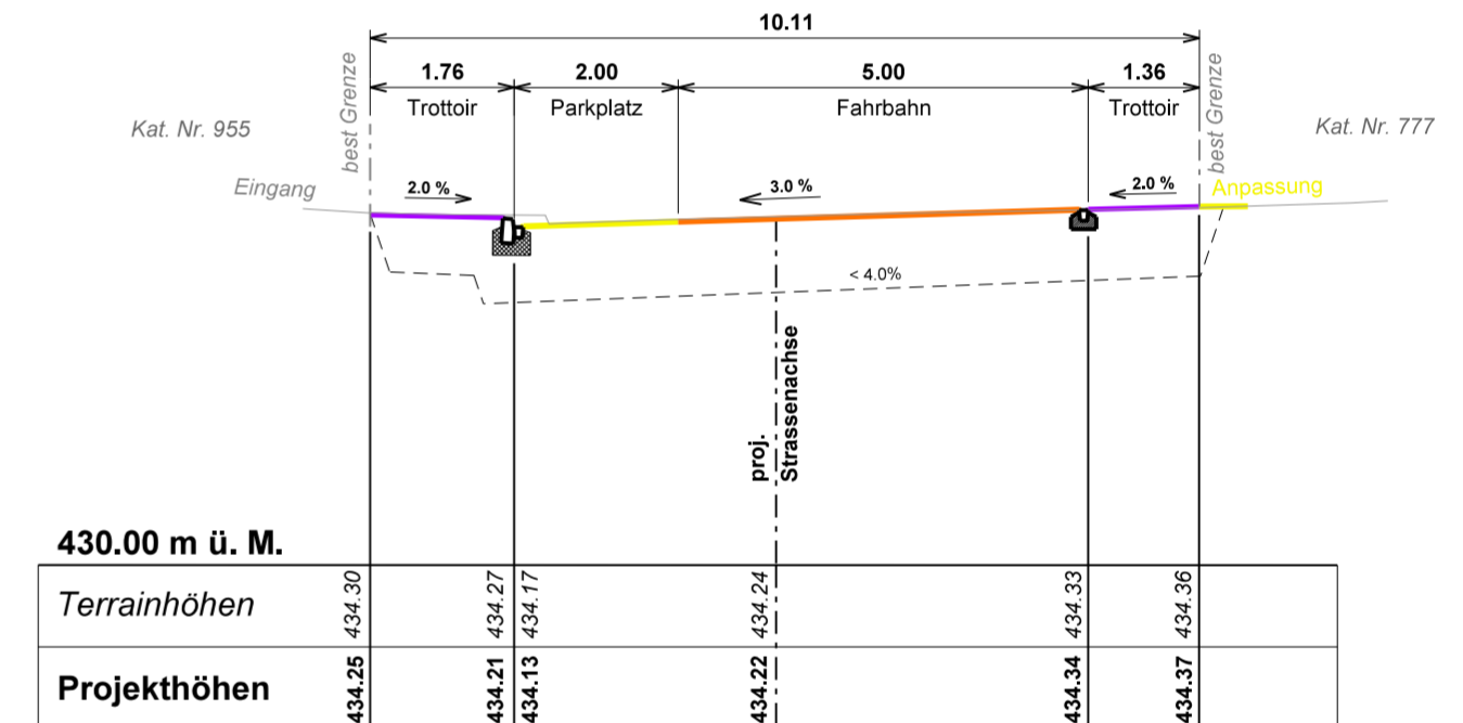
Profil 9 120.00m
