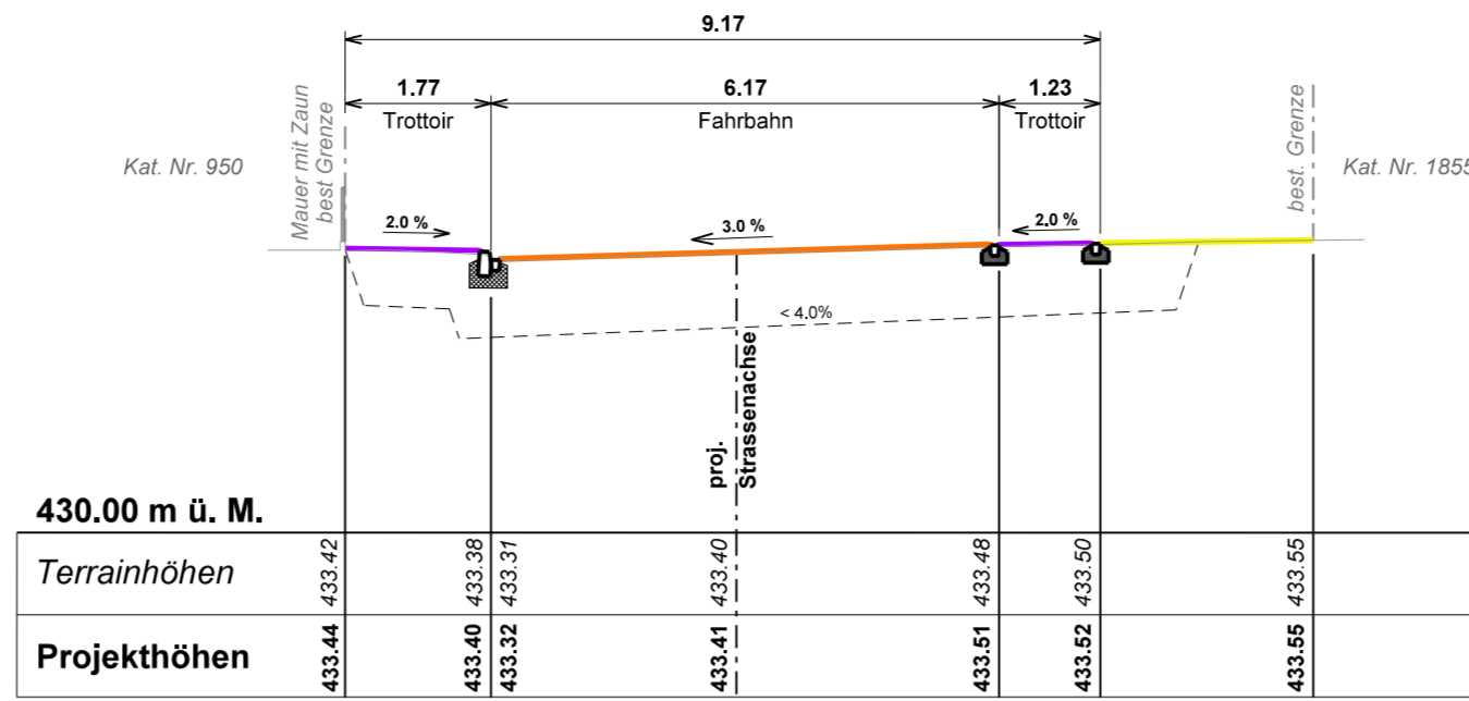
Profil 2 8.00m
