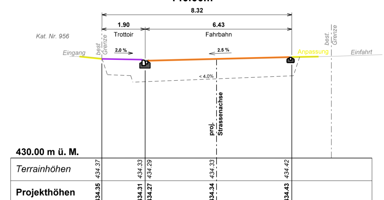
Profil 10 140.00m
