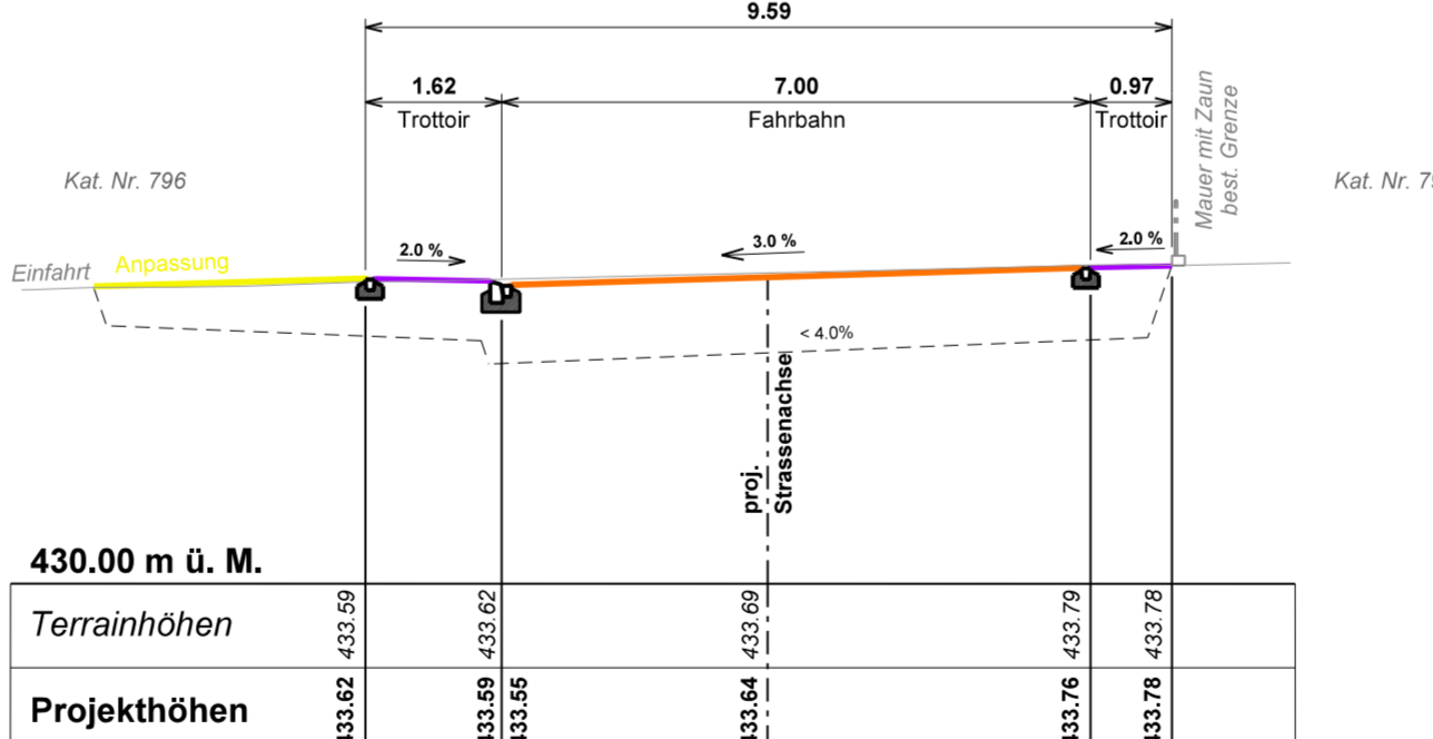
Profil 5 45.00m
