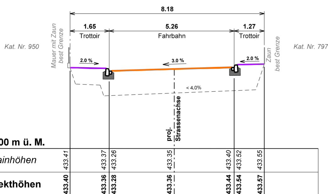
Profil 1 00.00m
