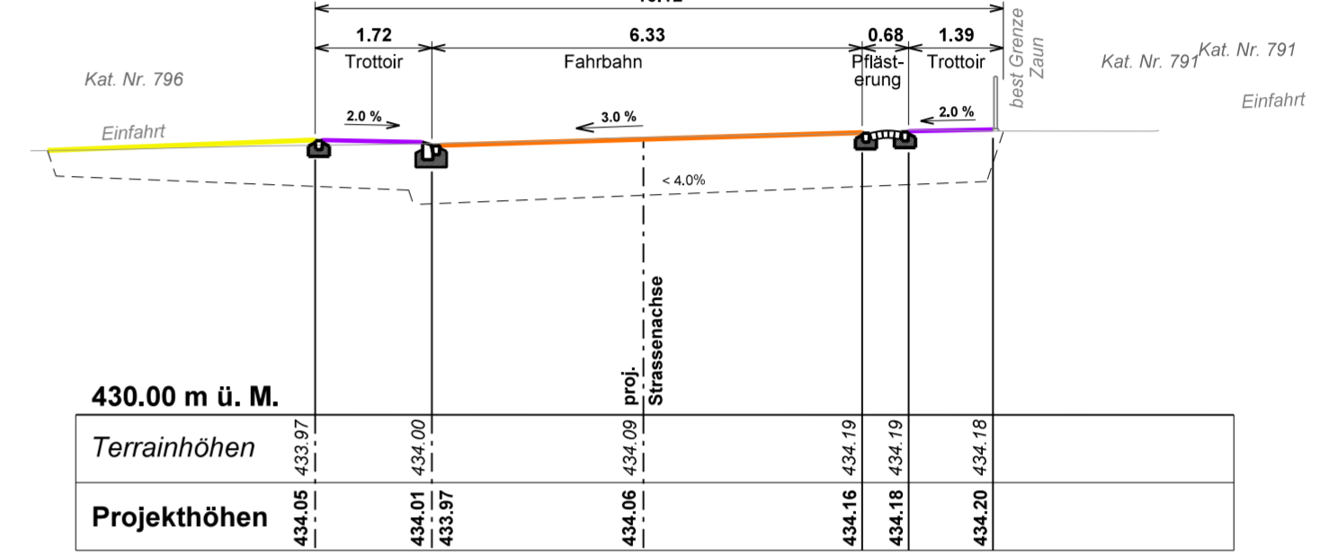
Profil 8 100.00m
