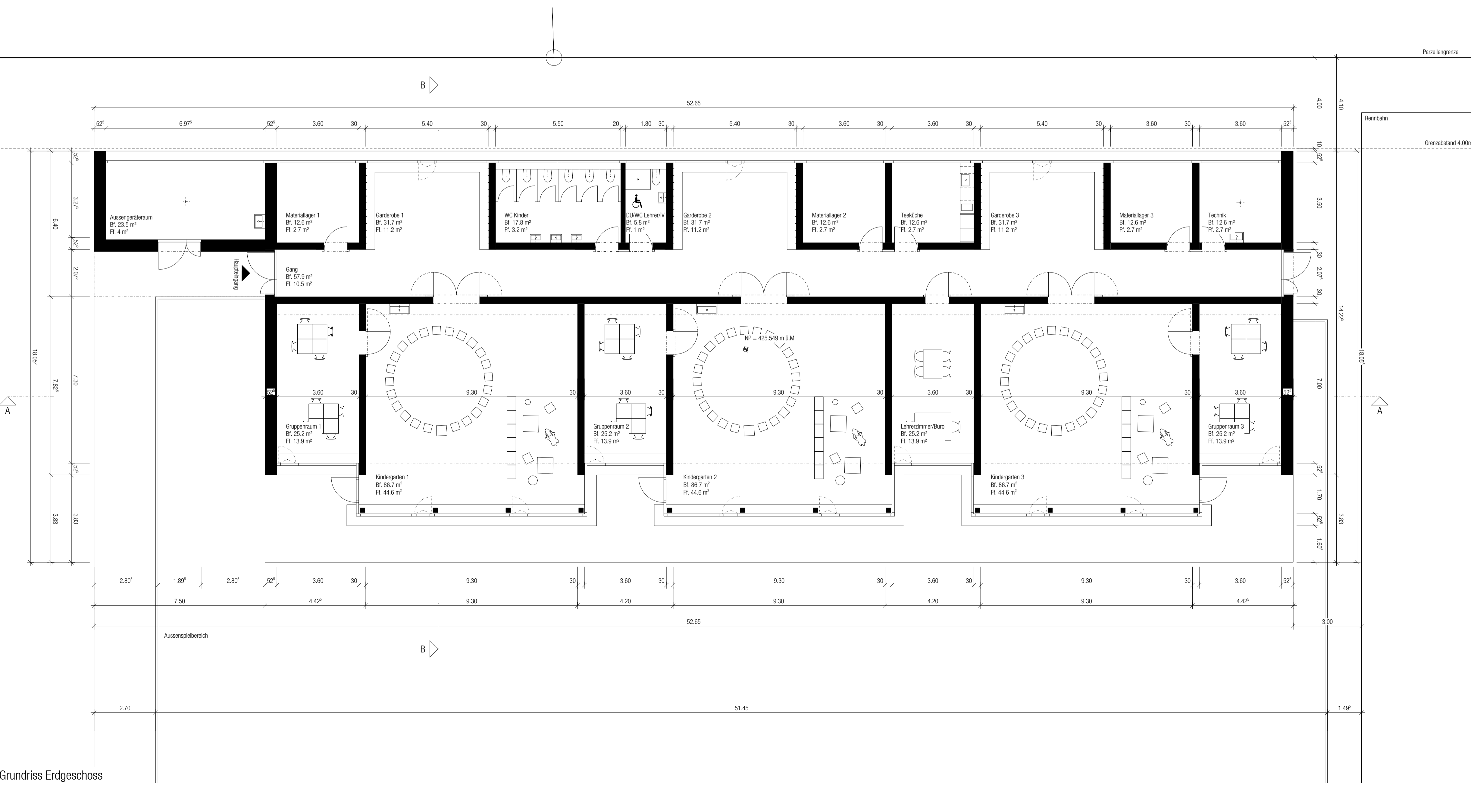
Grundriss Erdgeschoss
