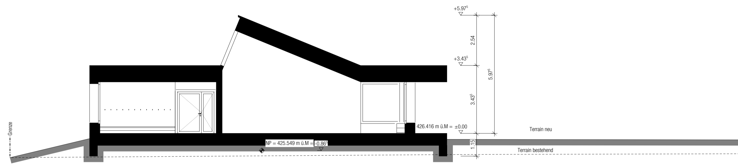
Gebäudeschnitt B - B
