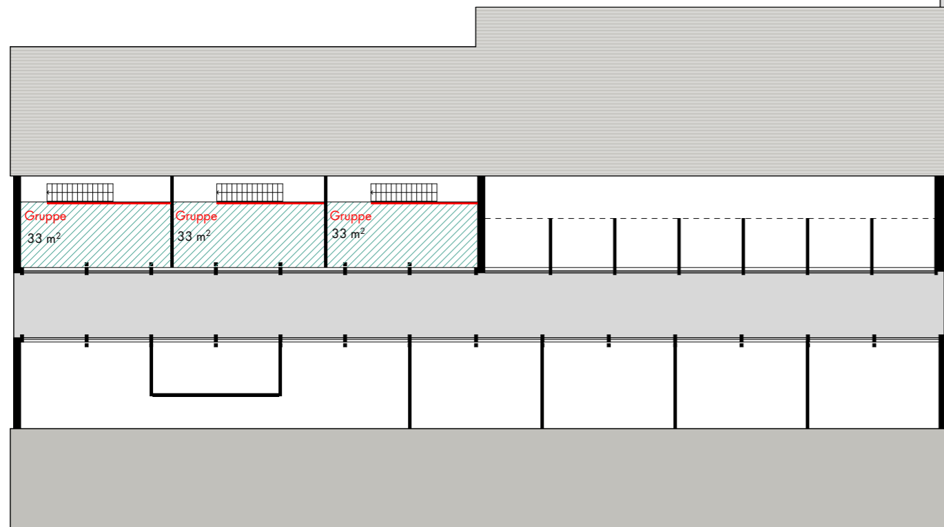
Galeriegesschoss 1/300
