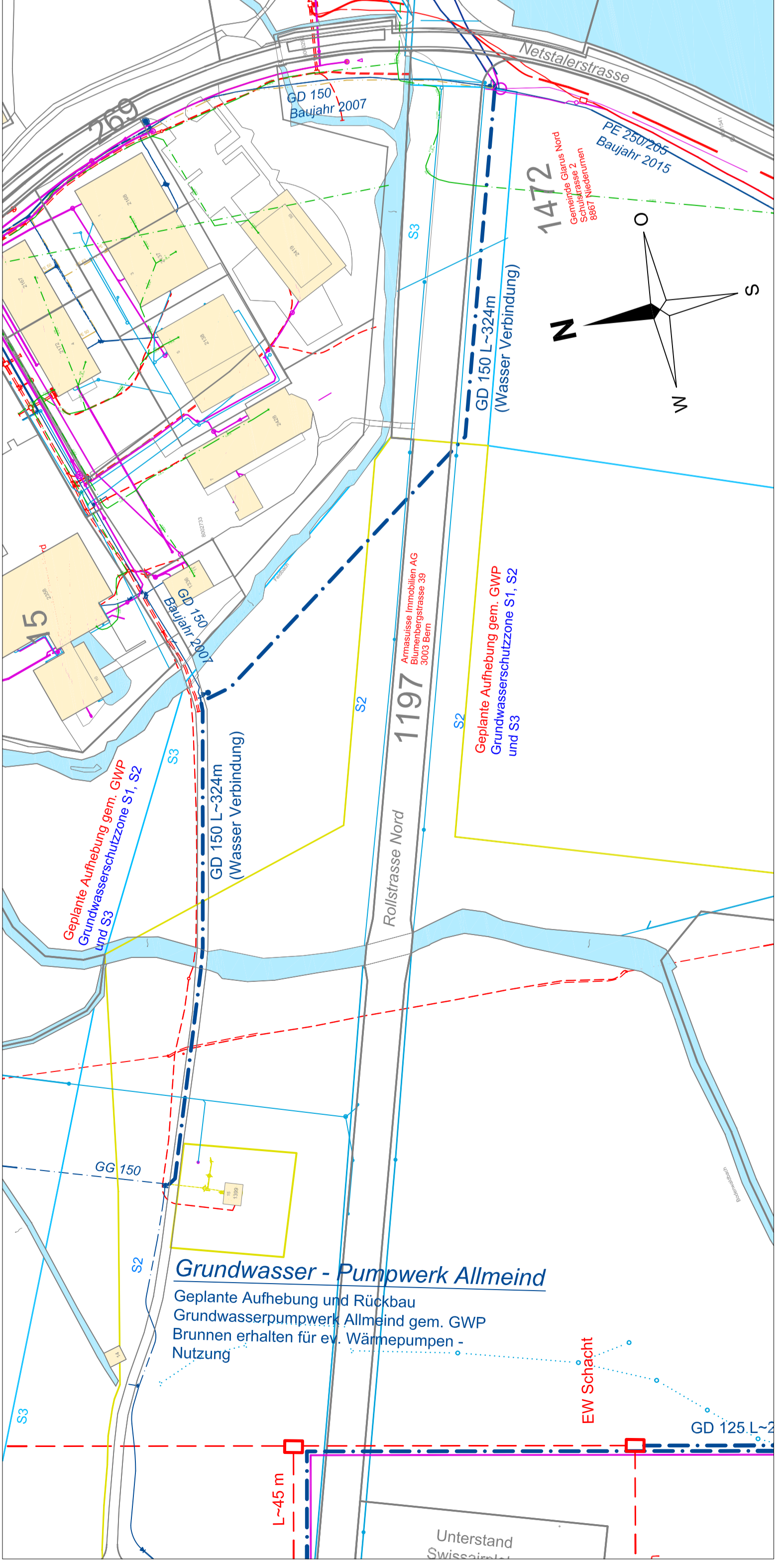
Ausschnitt Aufhebung PW Allmeind und Verbindung 1:1000 PW Allmeind bis Netstalerstrasse
