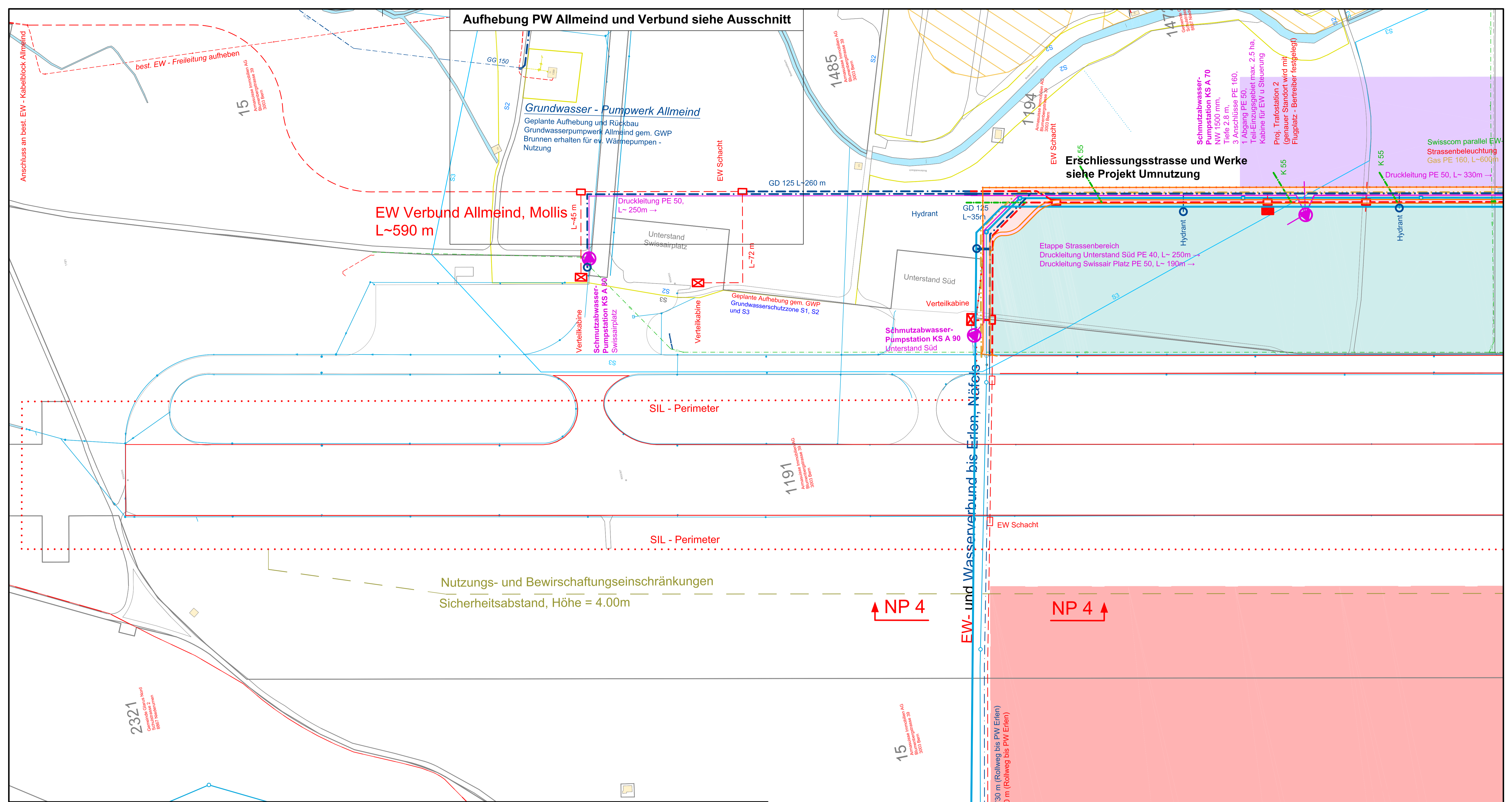
Ausschnitt Aufhebung PW Allmeind und Verbindung 1:1000 PW Allmeind bis Netstalerstrasse
